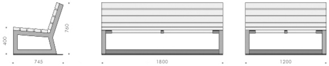
LB3/ LB2 Lehnenbank Dreisitzer/ Zweisitzer
