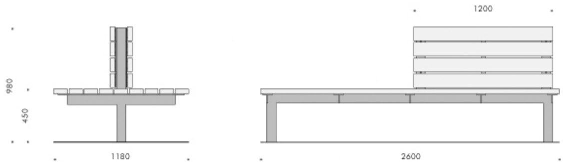
DL Doppelhockerbank mit Teillehne
