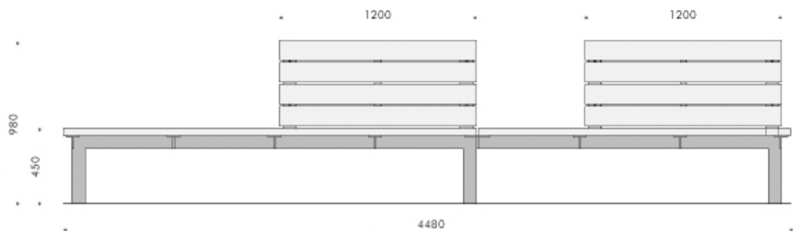
DL 448 lange Doppelhockerbank mit Teillehnen
